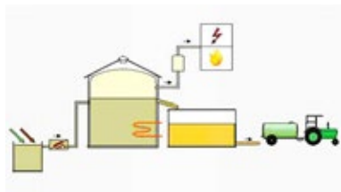
Figuur 13. Biogasinstallatie
