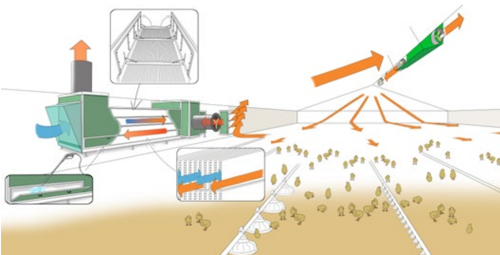
Figuur 18. Principe warmtewisselaar
