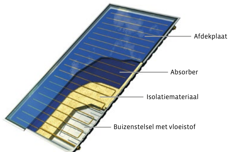
Figuur 11. Zonnecollector
