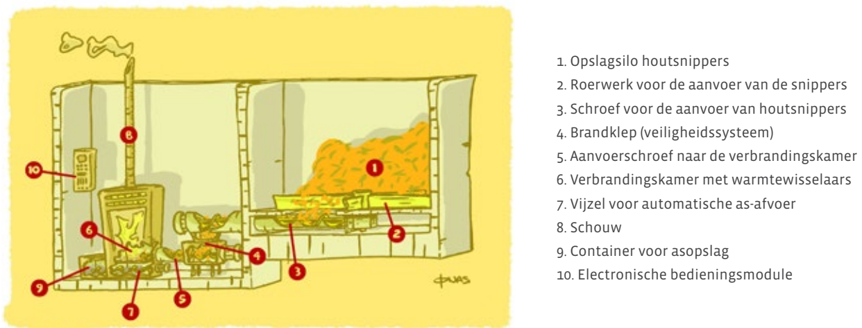
Figuur 15. Opslag en verwerking van houtsnippers
