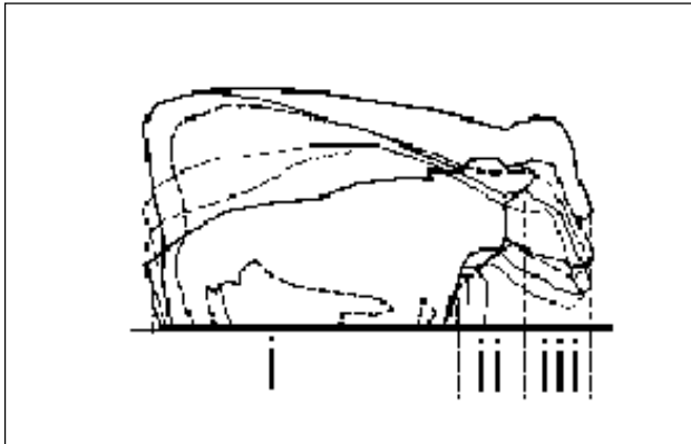
Figuur 17. De drie zones die de maten en het ontwerp van bindstanden en ligboxen bepalen
