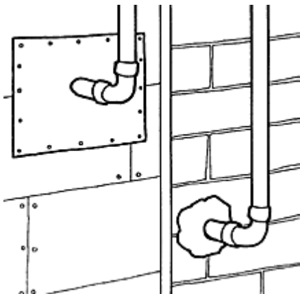
Figuur 4. Dichten van openingen rond leidingen
